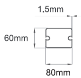
④ terminale
