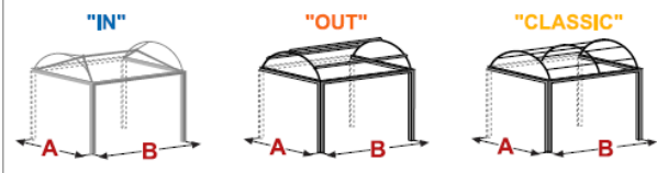
STRUTTURA ACCOPPIATA LATO A
