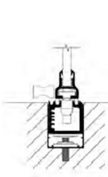
PROFILO INFERIORE INCASSATO CON COMPENSATORE
