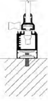
PROFILO INFERIORE CON COMPENSATORE
