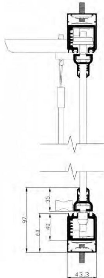
SEZIONE VERTICALE CON COMPENSATORE SUPERIORE E INFERIORE
